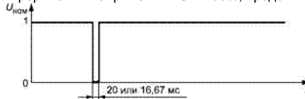
Рисунок В.2 - Прерывания напряжения \Delta U = 100\% , в течение одного цикла при номинальной частоте
