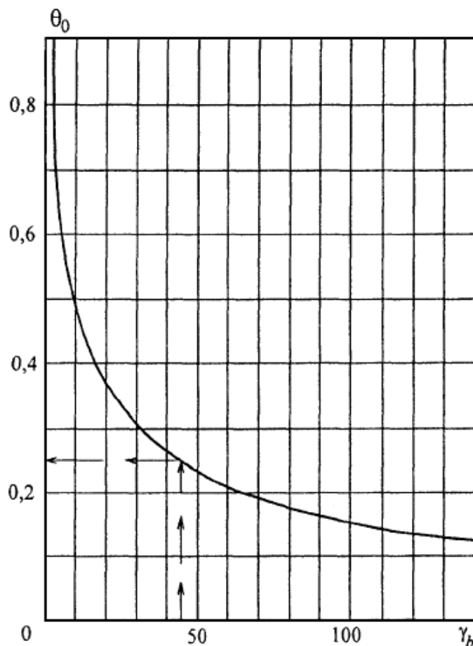
Рисунок М.1 - График для определения \theta_0
