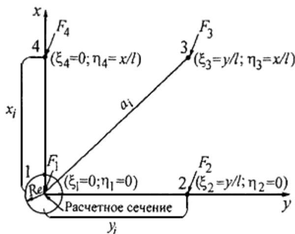
Рисунок 7.2 - Расчетная схема параметров загрузки опор воздушного судна
