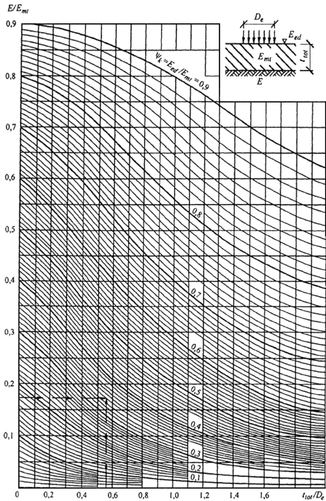
Рисунок К.4 - Номограмма для определения коэффициента \Psi_k
