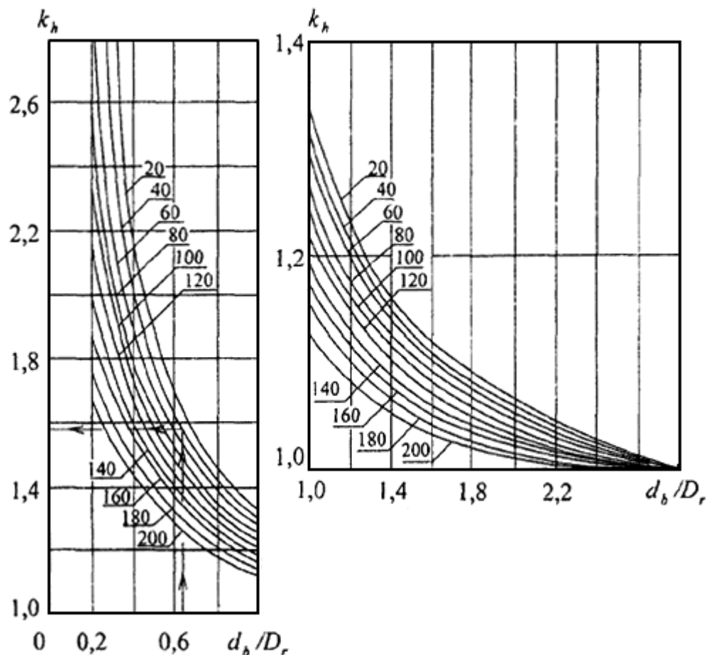
Рисунок Г.1 - График для определения коэффициента k_h жесткого массива.
