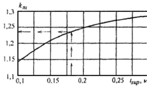
Рисунок К.3 - График для определения поправочного коэффициента k_m при расчете толщины усиления бетонного покрытия
