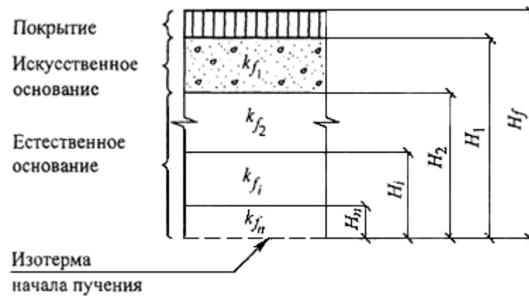
Рисунок Е.1 - Расчетная схема слоистого основания
