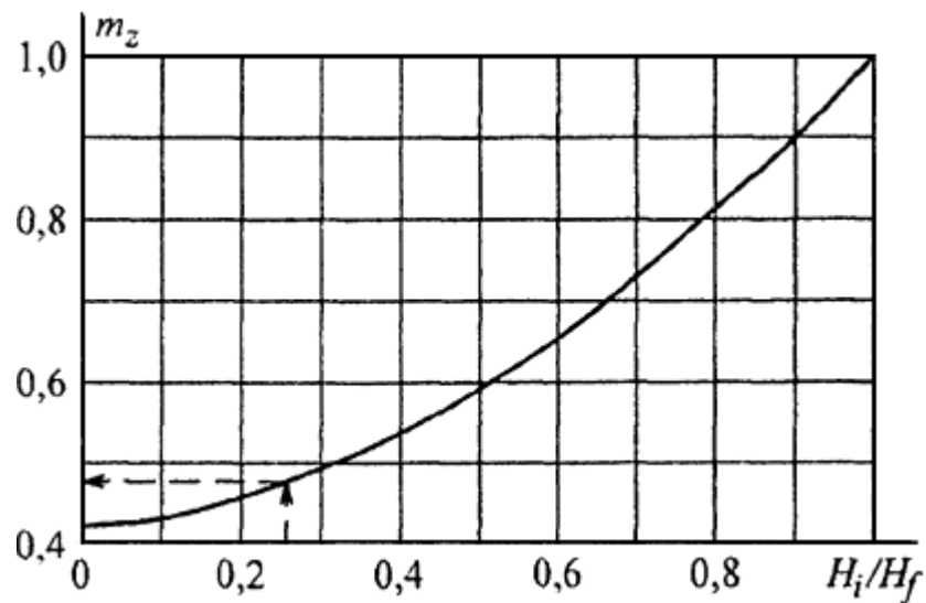
Рисунок Е.2 - График для определения коэффициента m_z
