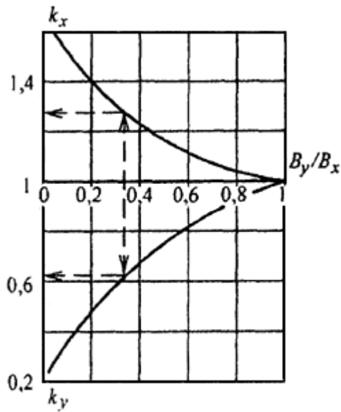
Рисунок К.2 - График для определения коэффициентов k_x и k_y , учитывающих перераспределение внутренних усилий в ортотропных плитах
