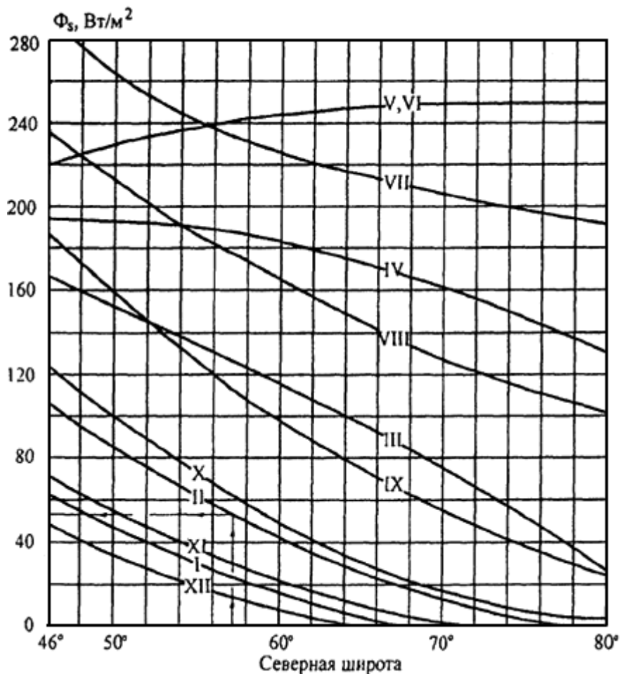
Рисунок Д.1 - Зависимость суммарной солнечной радиации \Phi_s от северной широты (I, II-XII - месяцы года)
