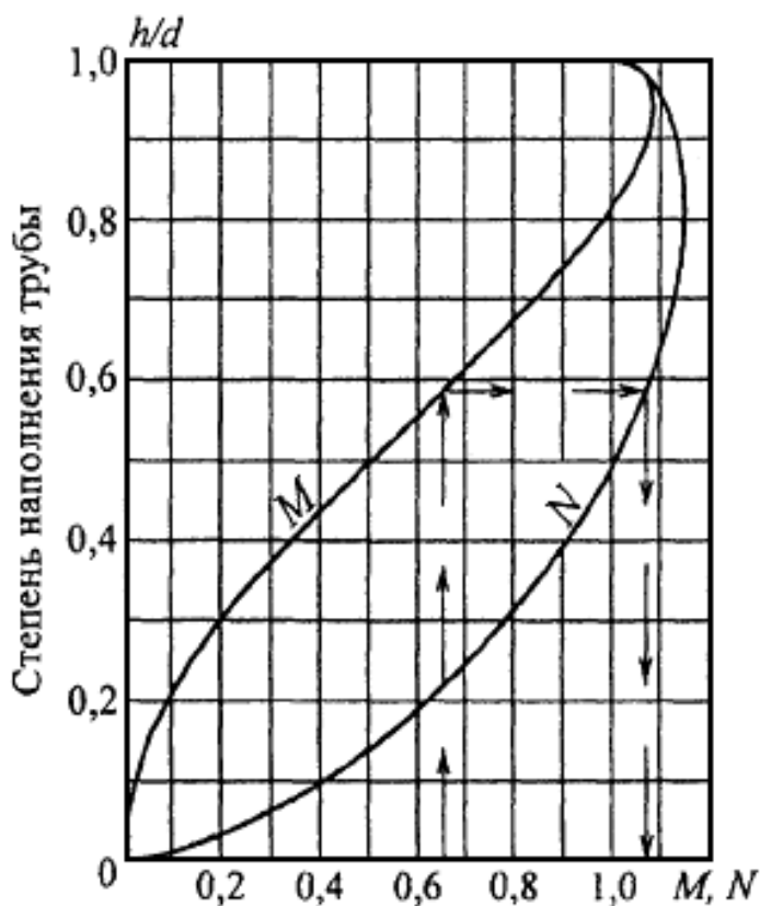
Рисунок Н.1 - График для определения коэффициента N и степени наполнения трубы (отношения глубины потока h к диаметру трубы d )
