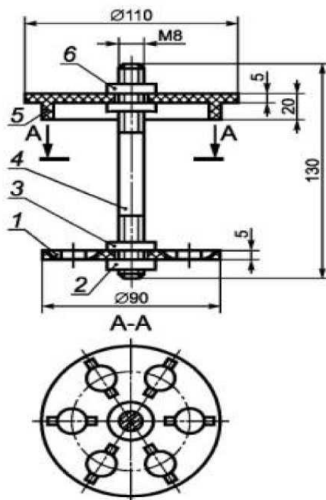
1 - кассета; 2, 3, 6 - специальная гайка; 4 - стержень; 5 - крышка Рисунок А.1
