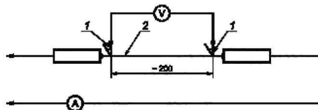
Рисунок А.1 — Схема испытательной цепи для калибровки проволоки нагревателя
