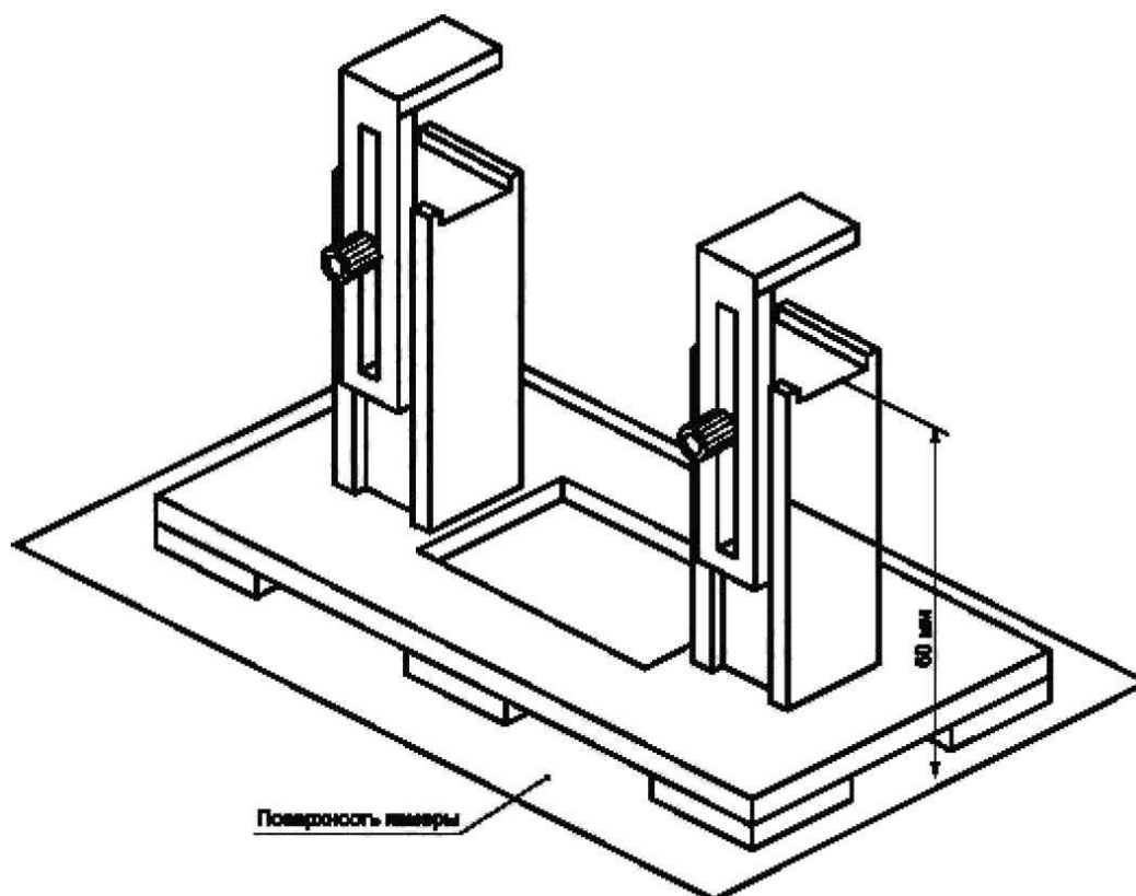
Рисунок 3 — Пример зажимного приспособления
