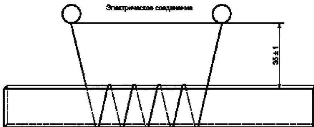
Рисунок 2 — Пример намотки проволоки на испытуемый образец
