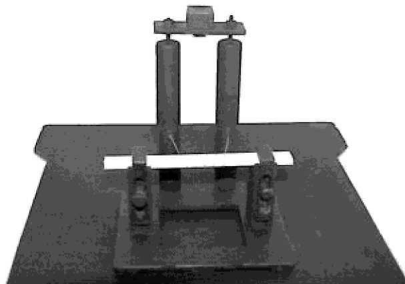
Рисунок 1 — Пример монтажа испытательного зажимного приспособления
