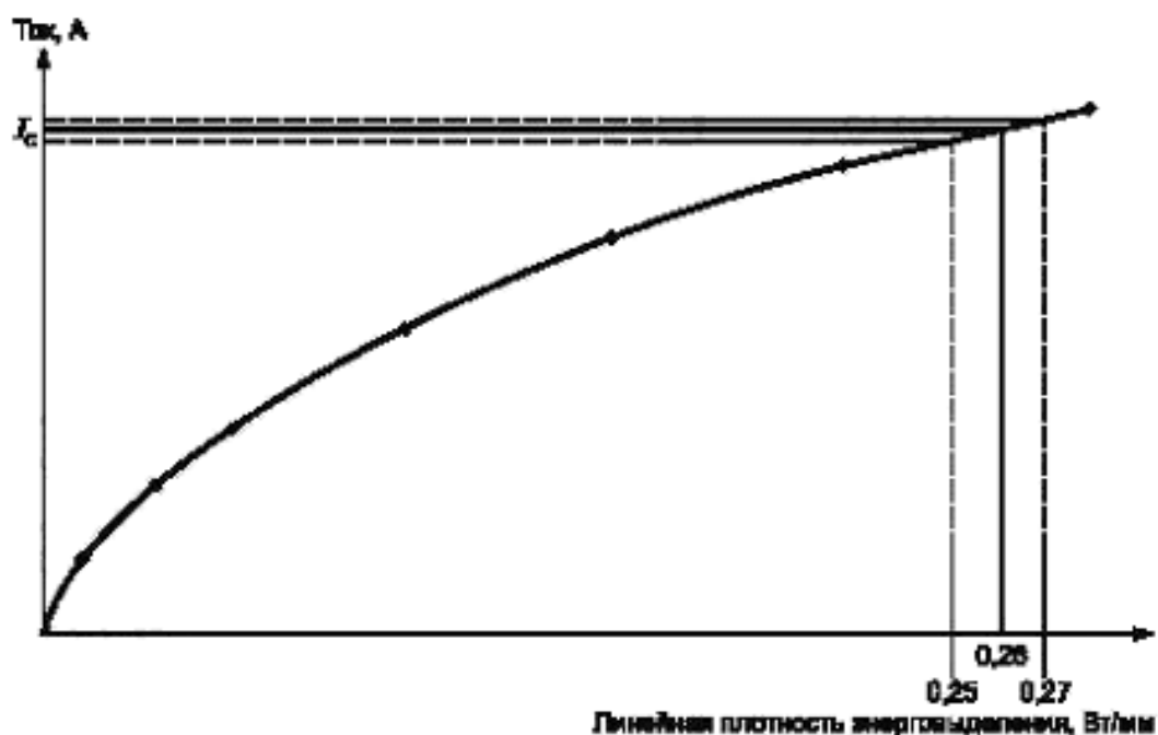
Рисунок А.2 — Калибровочная кривая
