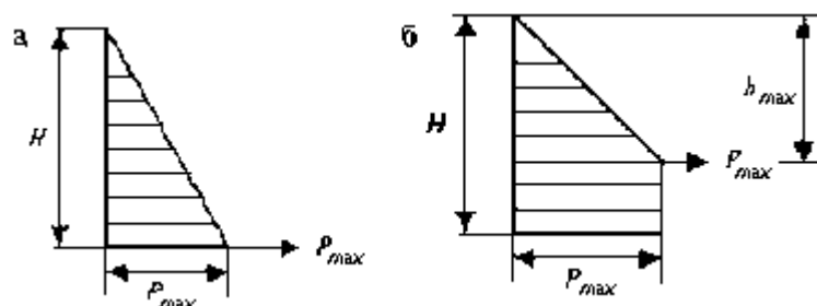
Рисунок 16.1 Расчетные эпюры бокового давления бетонной смеси а - гидростатическое давление; б - расчетное давление при уплотнении смеси внутренними вибраторами
