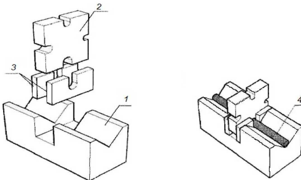
а) Поэлементно 1 - держатель; 2 - верхний нож; 3 - нижние ножи; 4 - опытный образец Рисунок Г.1 - Приспособление для испытания образцов на поперечный срез
