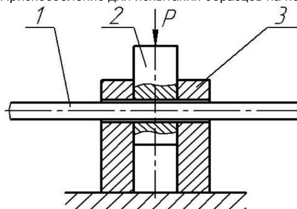
1 - опытный образец; 2 - верхний нож; 3 - нижние ножи Рисунок Г.2 - Схема приспособления с проходными отверстиями
