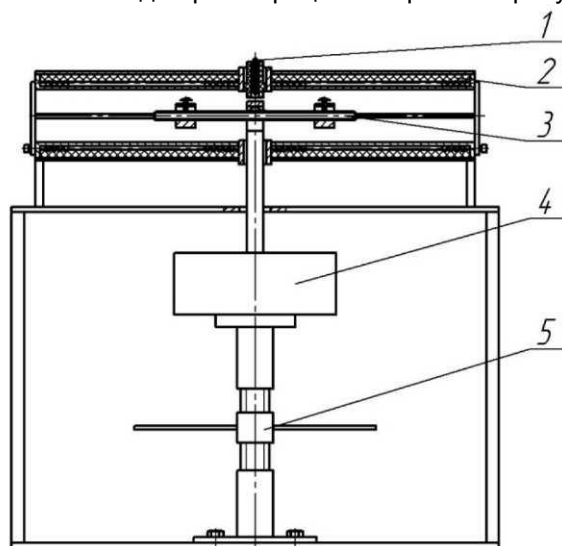
1 - датчик измерения температуры; 2 - нагревательная камера; 3 - образец; 4 - датчик измерения силы; 5 - нагружающий механизм
