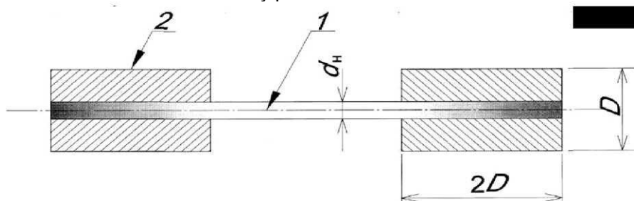
Рисунок В.1 - Схема образца для испытаний
