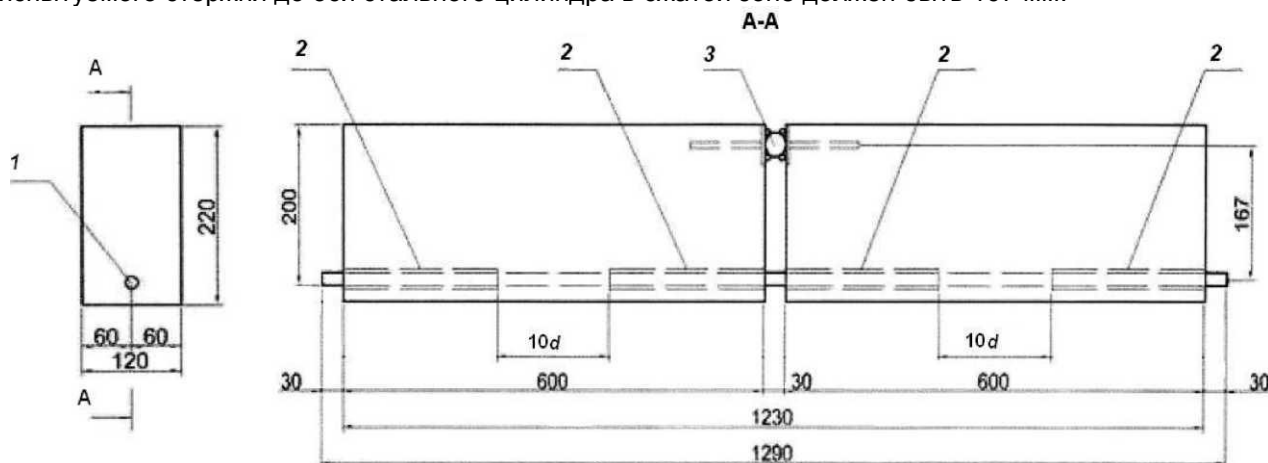
Рисунок Д.2 - Схема установки АКП в бетон при испытаниях балки на изгиб
