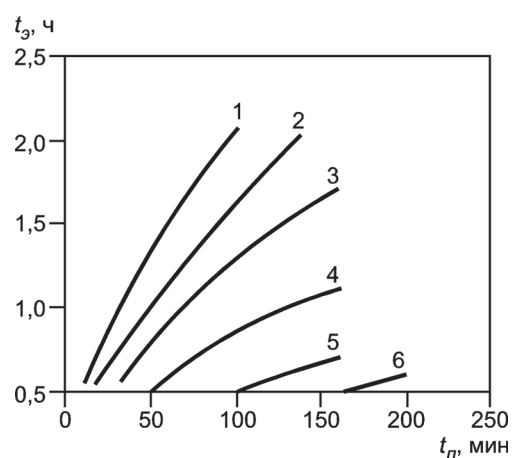
Рисунок Р.4 — Зависимость эквивалентной продолжительности пожара t_{\text{э}} от продолжительности пожара t_{\text{л}} для железобетонных и огнезащищенных металлических конструкций перекрытия при горении ЛВЖ и ГЖ
