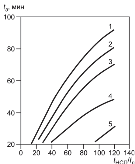
Рисунок Р.3 — Зависимость эквивалентной продолжительности пожара t_{\text{э}} от продолжительности пожара для железобетонных и огнезащищенных металлических конструкций перекрытия в условиях локальных пожаров t_{\text{л}} (или продолжительности НСП t_{\text{НСП}} ) при горении твердых и трудногорючих материалов
