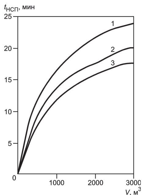
Рисунок Р.2 — Зависимость минимальной продолжительности начальной стадии пожара ( t_{\text{НСП}} ) от объема V и высоты H помещения
