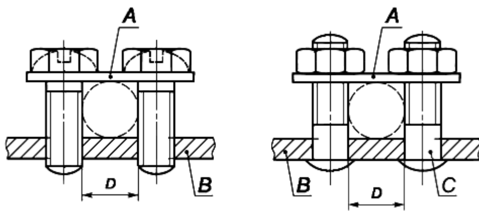
Рисунок F.2 - Пример винтовых и штыревых выводов
