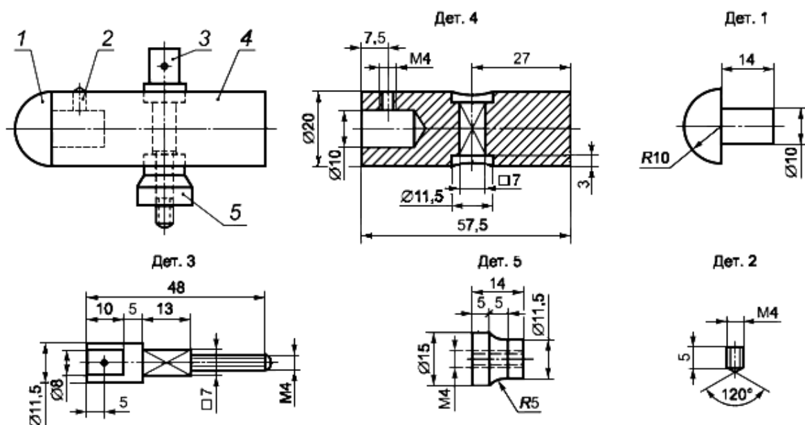
Рисунок 10 - Устройство для испытания на механический удар (см. 9.13.2)
