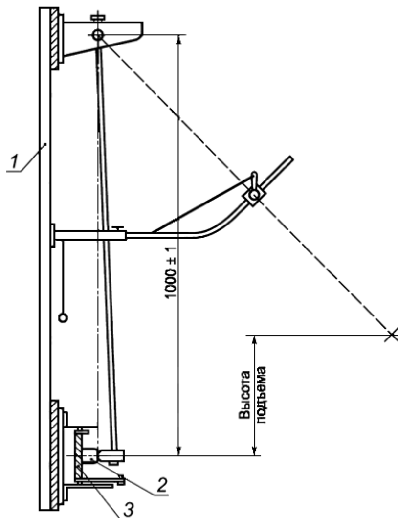
Рисунок 10 - Устройство для испытания на механический удар (см. 9.13.2)
