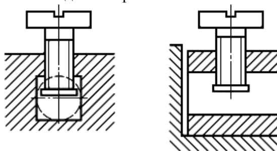
Выводы без прижимных пластин
