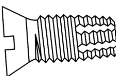
Рисунок 2 - Самонарезающий режущий винт (3.3.23)
