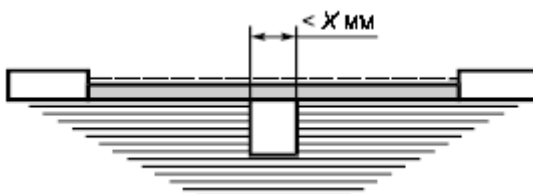
Рисунок F.1 - Размеры ребер
