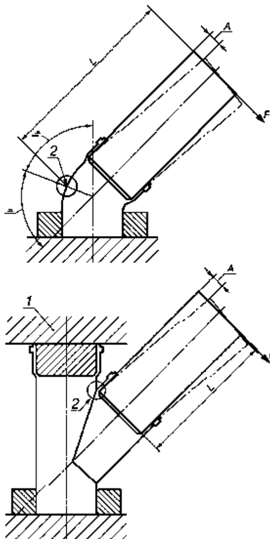
1 - фиксирующие элементы; 2 - зона возможного разрушения
