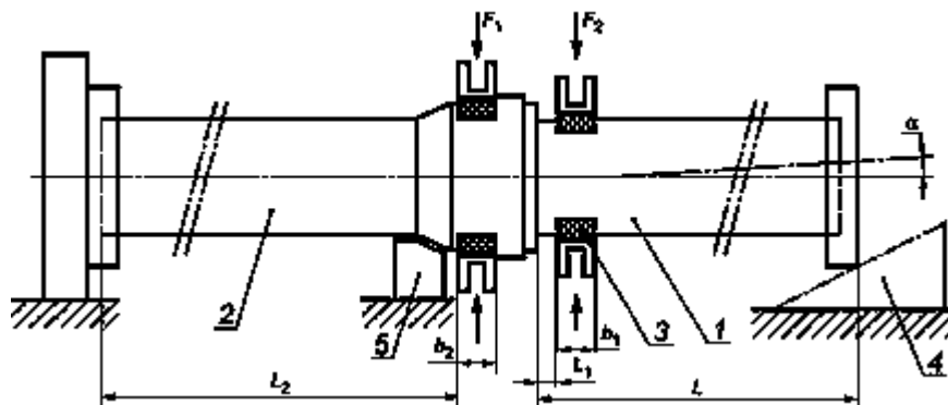
1 - труба; 2 - труба или фасонная часть с раструбом L_2 \geq 1000 мм; 3 - зажимы; 4 - регулируемая опора для создания осевого смещения; 5 - фиксатор раструба
