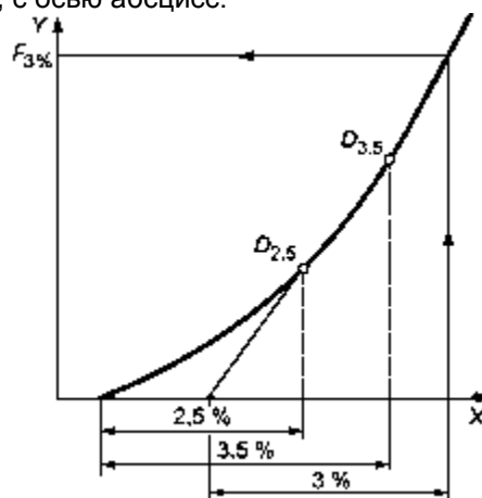
X - деформация у в процентах, Y - нагрузка F в ньютонах Рисунок 7
