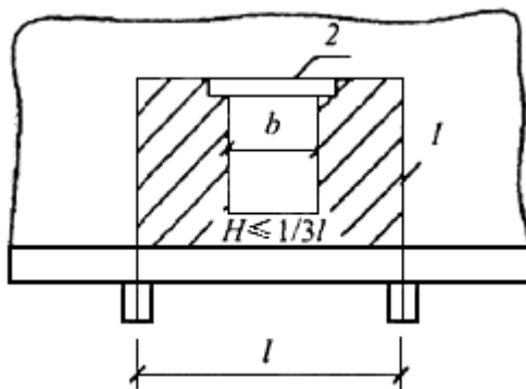
1 - нагрузка на рандбалку; 2 - железобетонная перемычка
