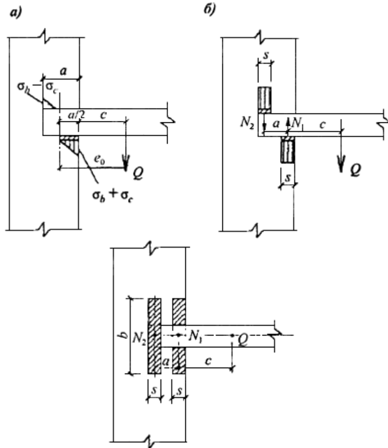
Рисунок 14 - Расчетные схемы заделки консольных балок
