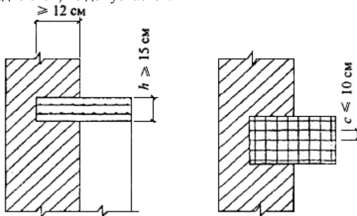
Рисунок 13 - Железобетонные распределительные плиты
