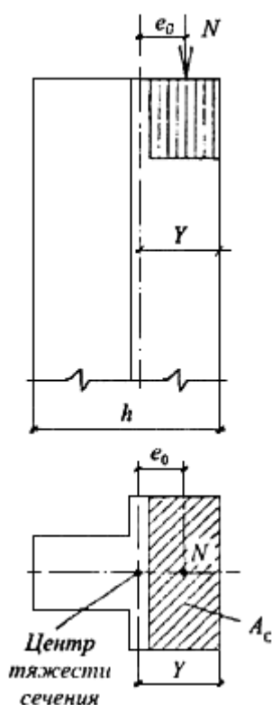
Рисунок 5 - Внецентренное сжатие
