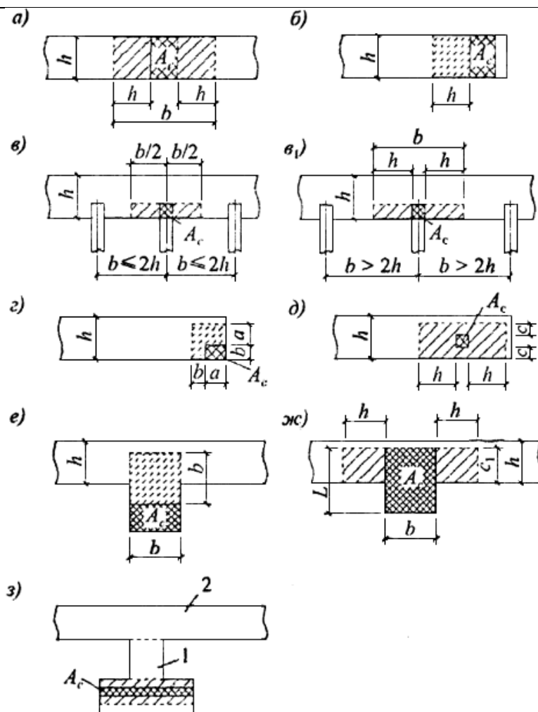
а-з - различные случаи местного сжатия
