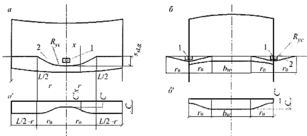
a - расположение источника замачивания под серединой (прогиб) здания; a' - схема изменения коэффициента жесткости при прогибе здания; b - расположение источников замачивания по торцам (выгиб) здания; b' - схема изменения коэффициента жесткости при выгибе здания; 1 - источники замачивания грунтов; 2 - кривые просадок грунта от собственного веса
