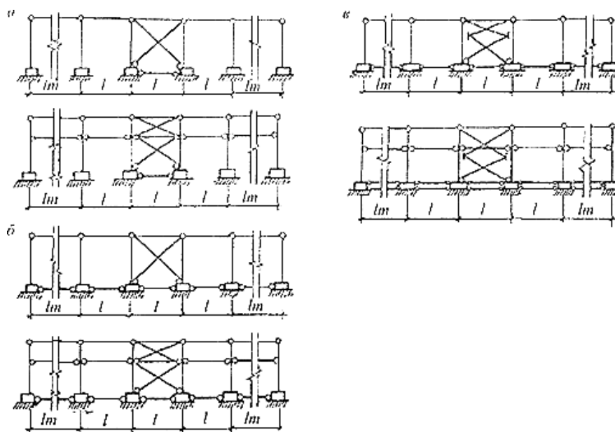
a-б - типы соединений элементов каркаса
