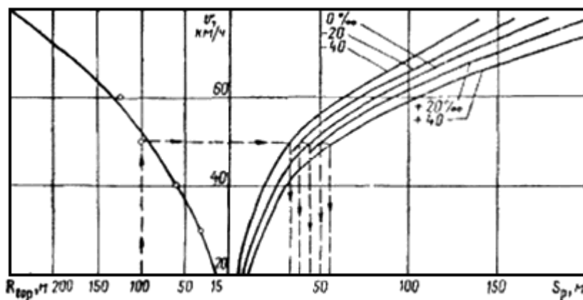
Рисунок 6.6 - График уменьшения длины полосы разгона при различных продольных уклонах в зависимости от радиуса сопряжения съездов Скорость движения, км/ч, на кривых в плане выражается формулой:
