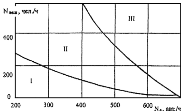
Рисунок 6.1 - Области применения пешеходных переходов различных типов
